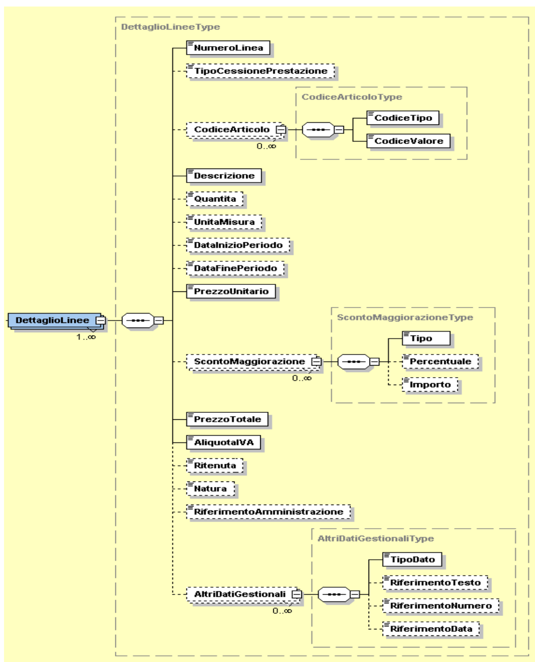
Figura 27: Elemento DettaglioLinee
