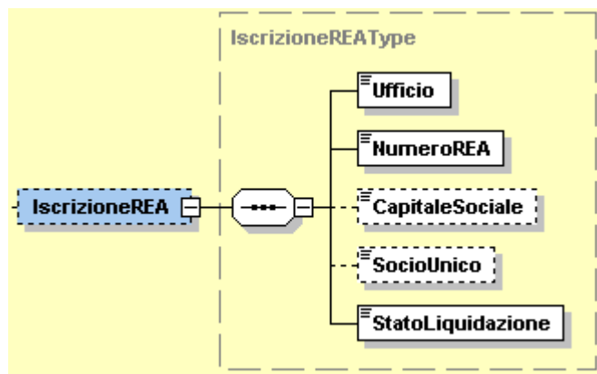
Figura 9: Elemento IscrizioneREA
