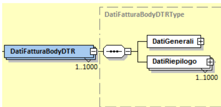
Figura 20 - Elemento DatiFatturaBodyDTR
