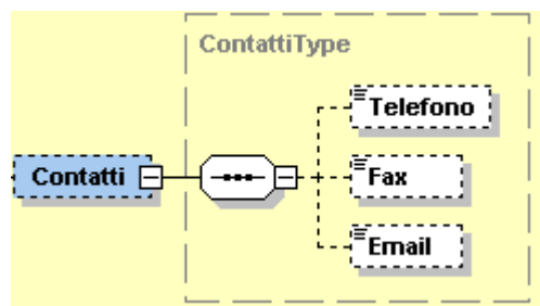
Figura 10: Elemento Contatti
